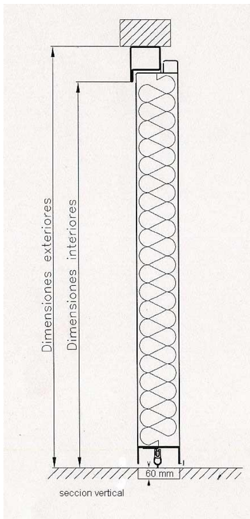
DETALLE BURLETE AUTOMÁTICO
